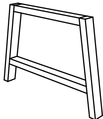
A-jalka, terästä 5x3
